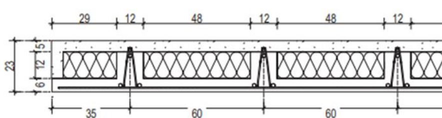
Figure : Coupe du plancher dalle BB complet. Epaisseur Dalle BB : 18 cm.
