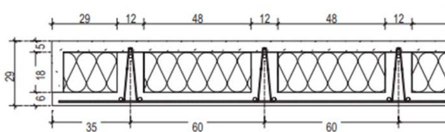
Figure : Coupe du plancher dalle BB complet. Epaisseur Dalle BB : 24 cm.
